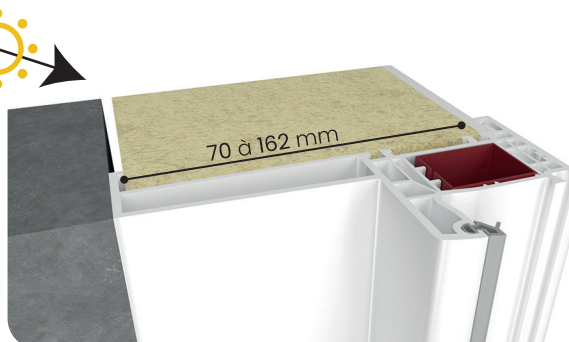
Dormant monobloc pour doublage de 70 à 162 mm réf 140x12 à 140x19
