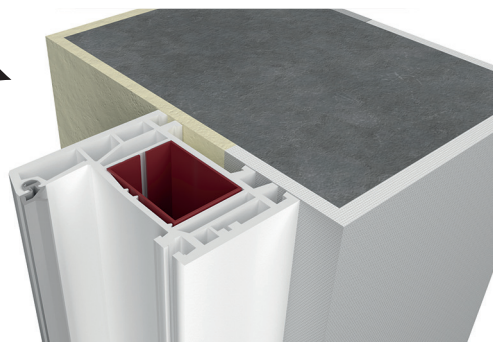
Dormant entre murs - réf 140x01
