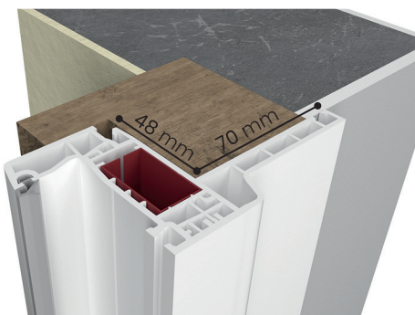
Dormant de rénovation aile de 70 mm avec éloignement de 22 mm pour dos de dormant 48 mm - réf 140x13
