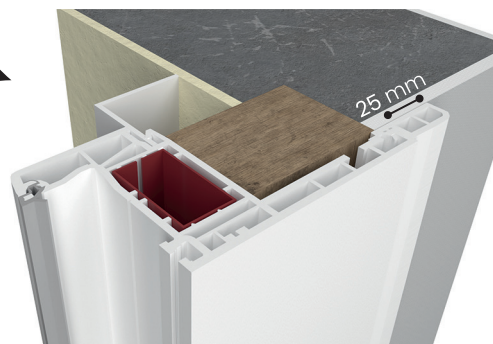
Elargisseur de recouvrement 25 mm réf 140x17 + 140279 (65 + 25 = CJ de 90)
